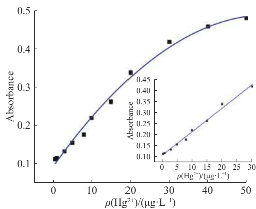
图6 \text{Hg}^{2+} 质量浓度与吸光度之间的关系
