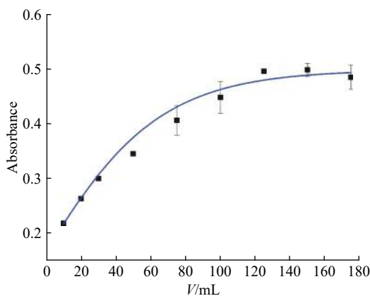
图3 样品体积对汞-双硫脲络合物吸光度的影响
