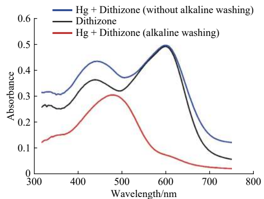
图5 富集双硫脲、汞-双硫脲络合物(碱洗/未碱洗)的膜固相光谱图
