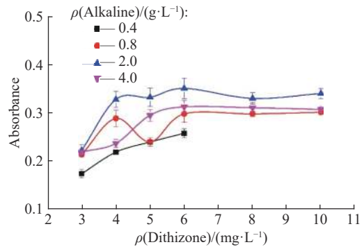
图4 碱和双硫脲质量浓度对汞-双硫脲络合物吸光度的影响
