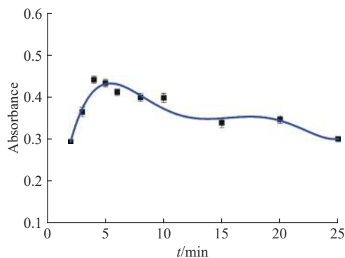
图 2 反应时间对汞-双硫脲络合物吸光度的影响
