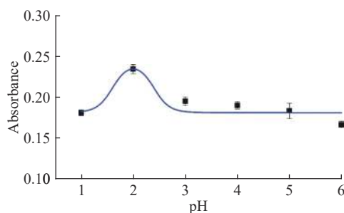
图 1 样品溶液 pH 值对汞-双硫脲络合物吸光度的影响
