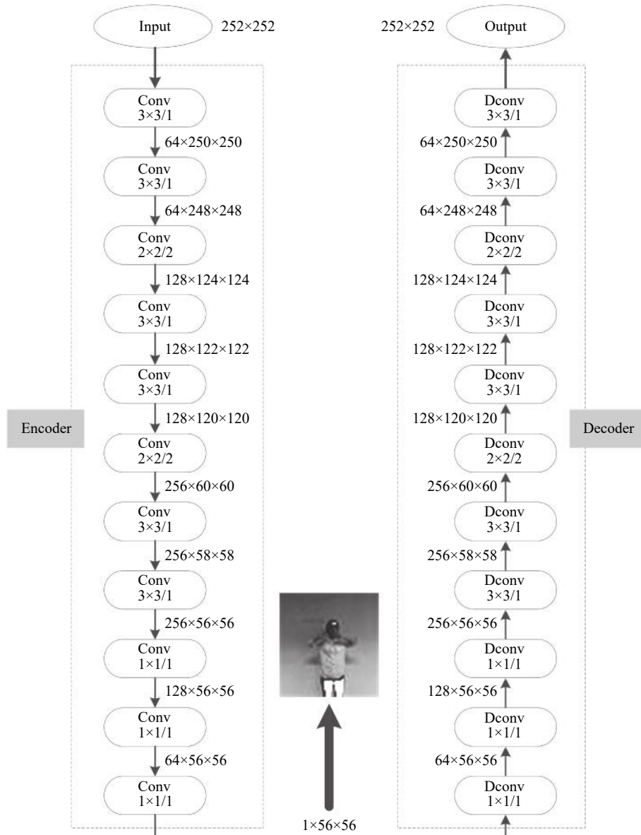
图2 用于特征提取的CAE网络结构
