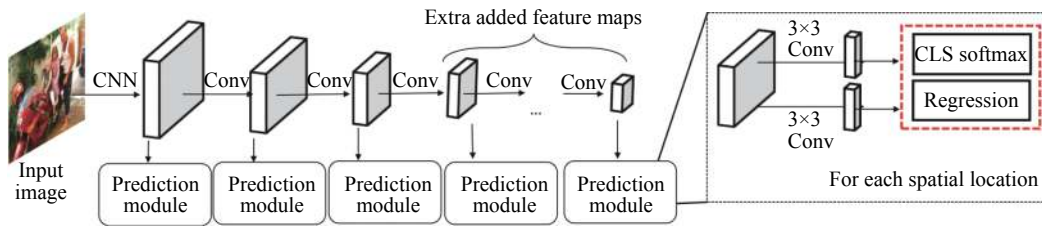
图 6 SSD 网络结构图 Fig. 6 Network structure of SSD
